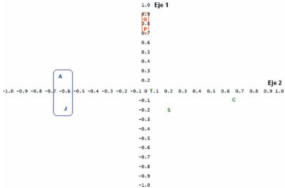
Figura 6. Grupos de factores (rojo y azul) en los dos primeros ejes en el ACP considerando los datos consolidados de los cuatro periodos de estudio en el OPC. Abundancia de quetognatos (A =adultos, J =juveniles), periodo del día (P), clorofila-a (C), salinidad (S) y temperatura (T)
