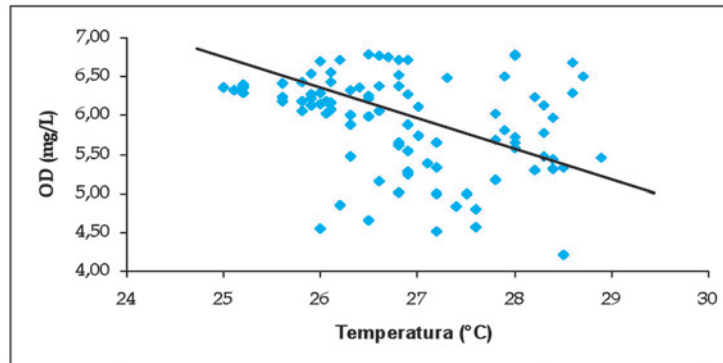
Figura 2. Gráfico de regresión entre datos de temperatura y OD para la Bahía de Tumaco durante 2008.
