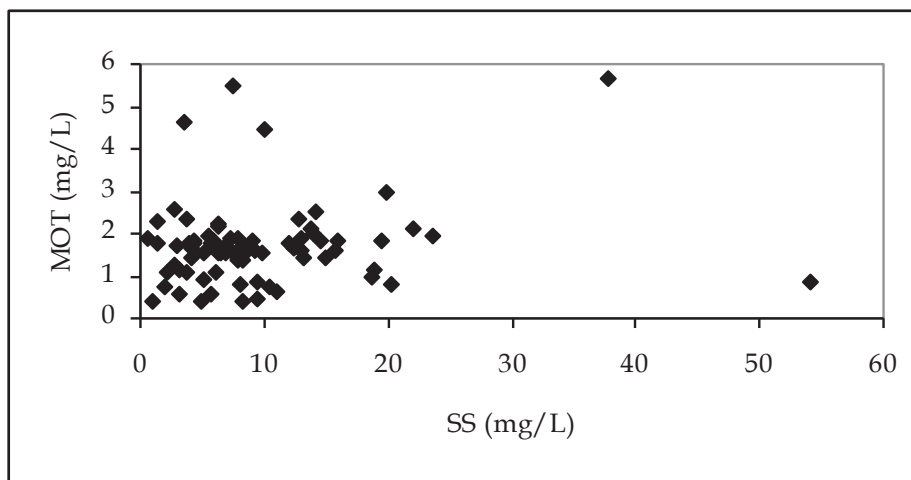
Figura 6. Gráfico de correlación de las concentraciones de materia orgánica total y sólidos en suspensión, determinadas entre 2007-2008.
