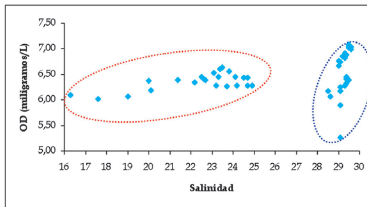
Figura 3. Diagrama de correlación entre concentraciones de OD y salinidad para la Bahía de Málaga. (•••) Resultados primer semestre, (•••) resultados segundo semestre.
