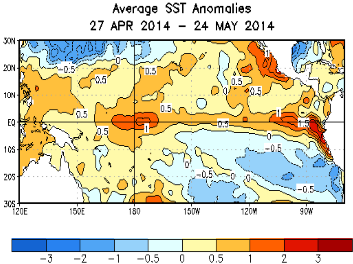
Figura 3. Anomalías de TSM en el pacifico tropical, promediadas del 27 de abril al 24 de mayo de 2014 (°C). (Fuente: Climate Prediction Center, NOAA).
