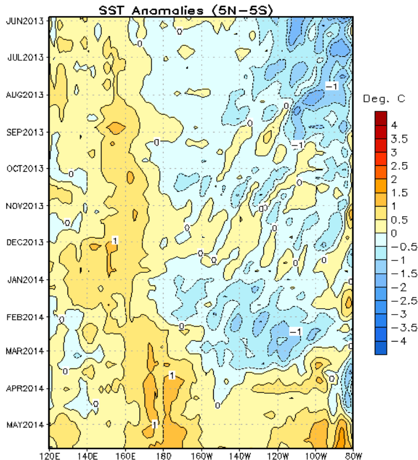
Figura 1. Evolución de la TSM en el Pacífico Ecuatorial (°C), entre 5°S y 5°N. (Fuente: Climate Prediction Center, NOAA).
