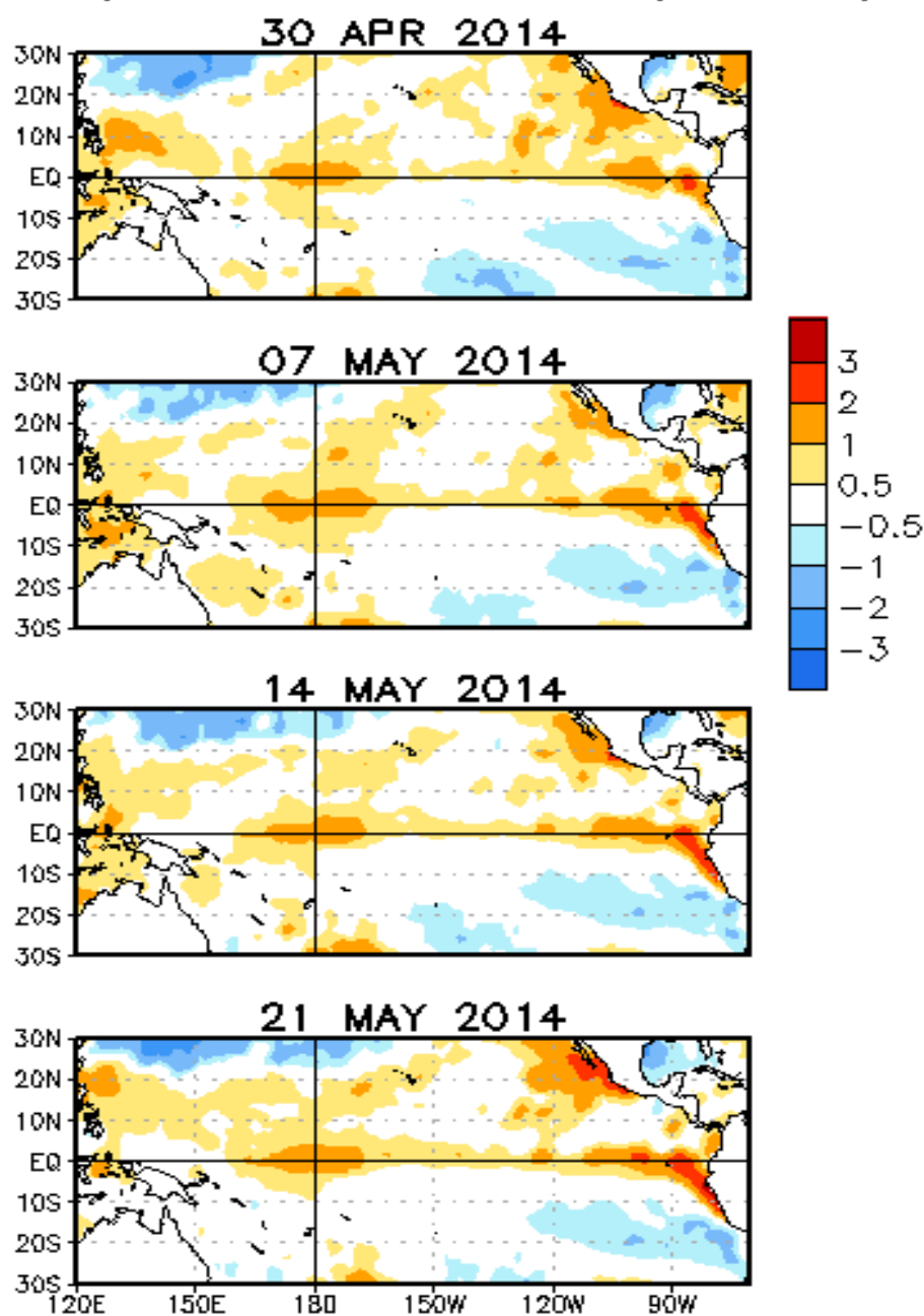
Figura 4. Anomalías de TSM para el Océano Pacífico durante las últimas cuatro semanas (°C). (Fuente: Climate Prediction Center, NOAA).
