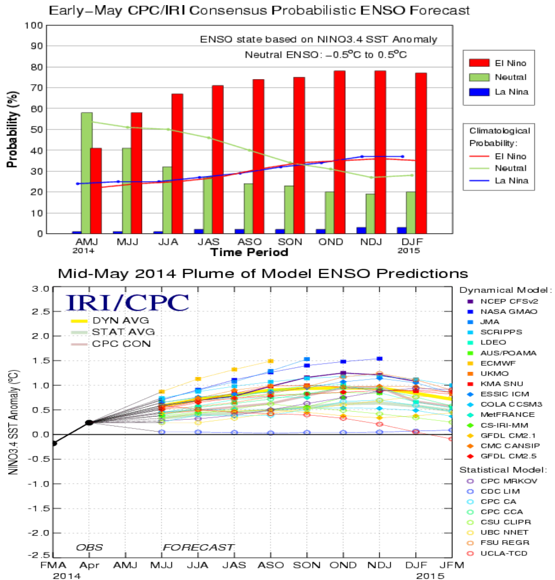
Figura 5. Pluma de salidas de los modelos estadísticos y dinámicos de predicción de condiciones ENOS abril 16 de 2014. (Fuente: IRI/CPC).
