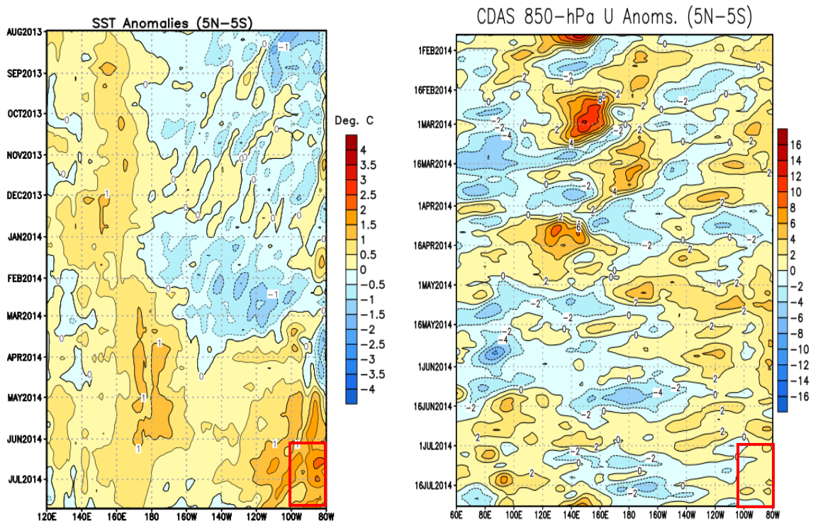
Figura 1. Evolución anomalías de la TSM y viento (componente U) en el Pacífico Ecuatorial (°C), entre 5°S y 5°N.
