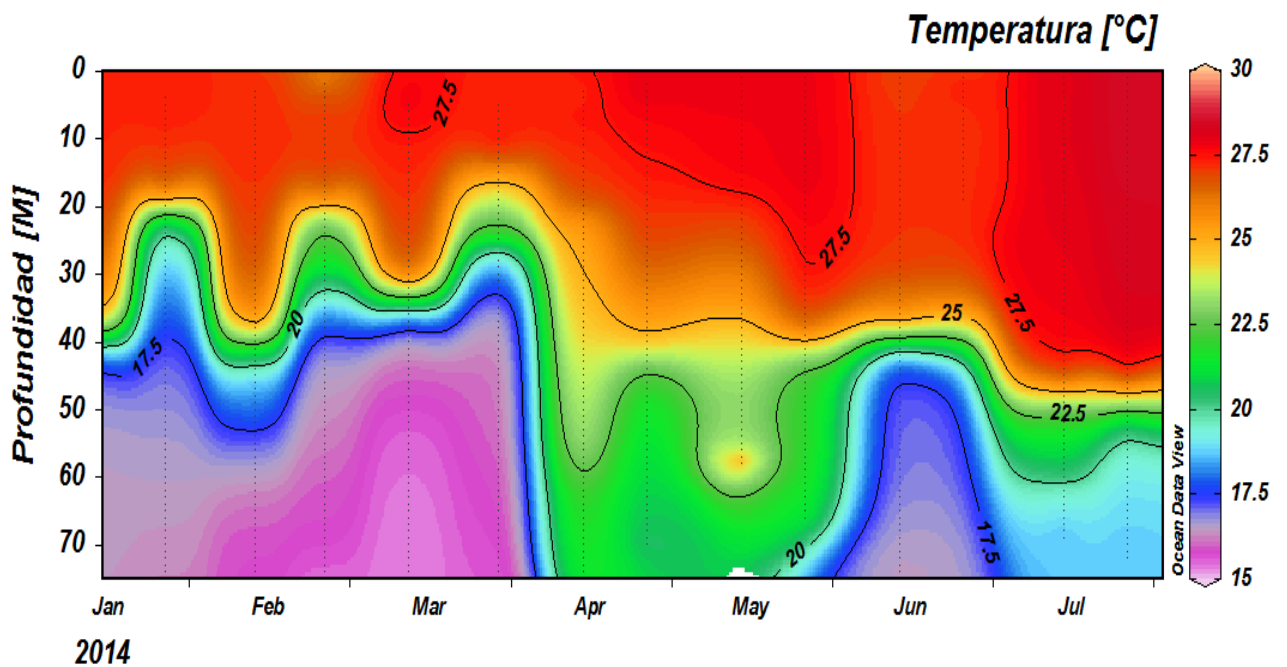
Figura 6. Serie temporal de temperatura del agua en la estación oceánica No. 5 entre 0 a 70 metros de profundidad. Período enero 2014 – Julio 2014 (°C) (Fuente: CCCP)
