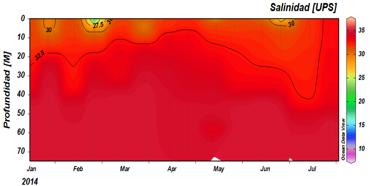
Figura 8. Serie temporal salinidad en la estación oceánica No. 5 entre 0 a 70 metros de profundidad. Período Enero 2014 – Julio 2014 (UPS) (Fuente: CCCP)
