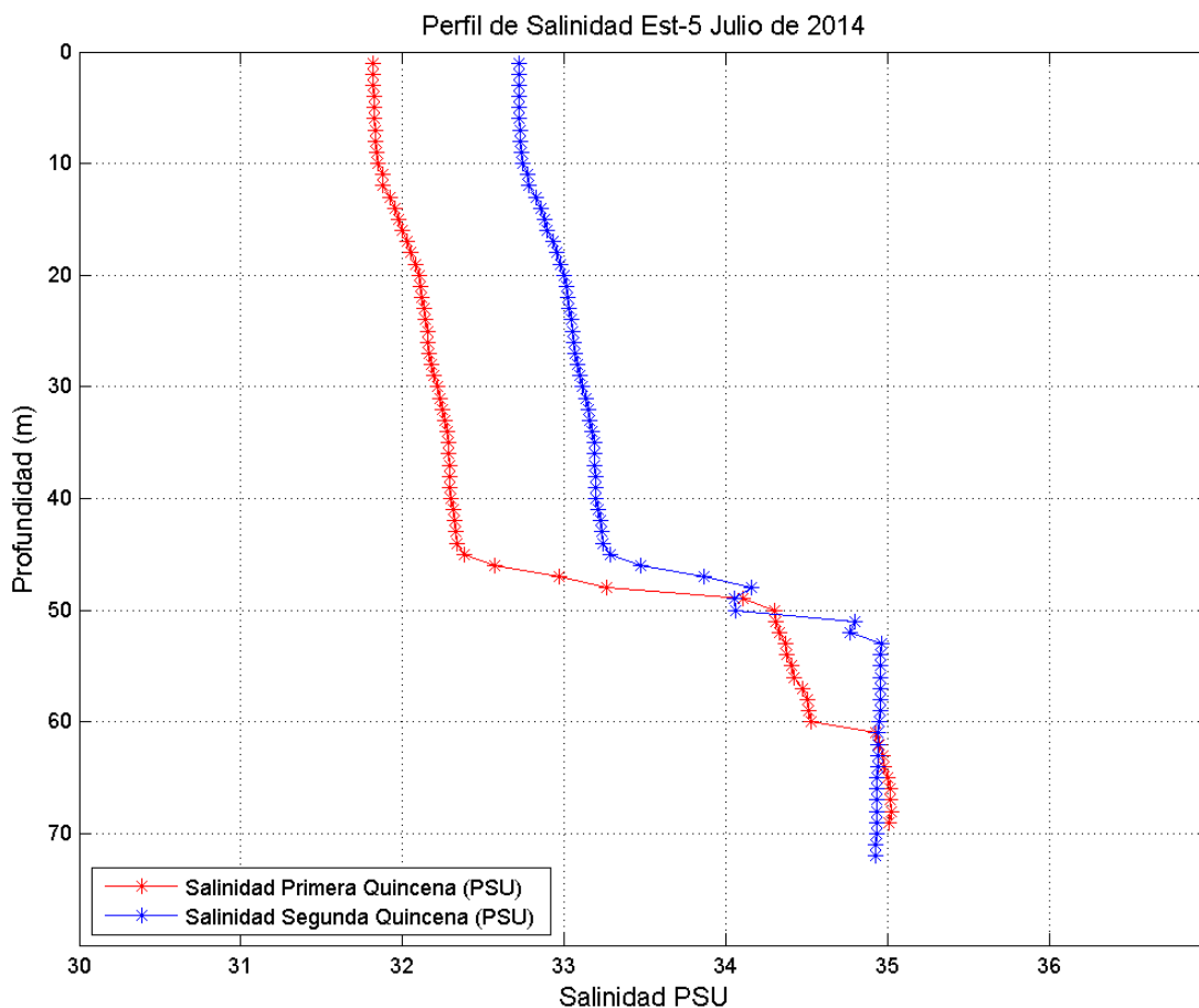
Figura 9. Perfil de la salinidad del agua durante el monitoreo del mes de Julio/14 en la “Estación No.5”. (Fuente: CCCP)
