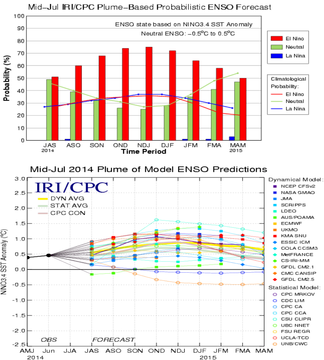
Figura 5. Pluma de salidas de los modelos estadísticos y dinámicos de predicción de condiciones ENOS julio 19 de 2014. (Fuente: IRI/CPC).
