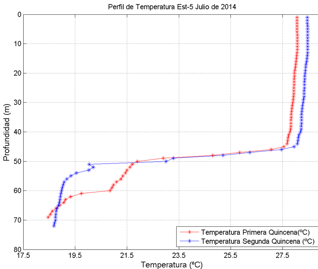
Figura 7. Perfil TSM durante el monitoreo del mes de Julio/14 en la “Estación No.5”.
