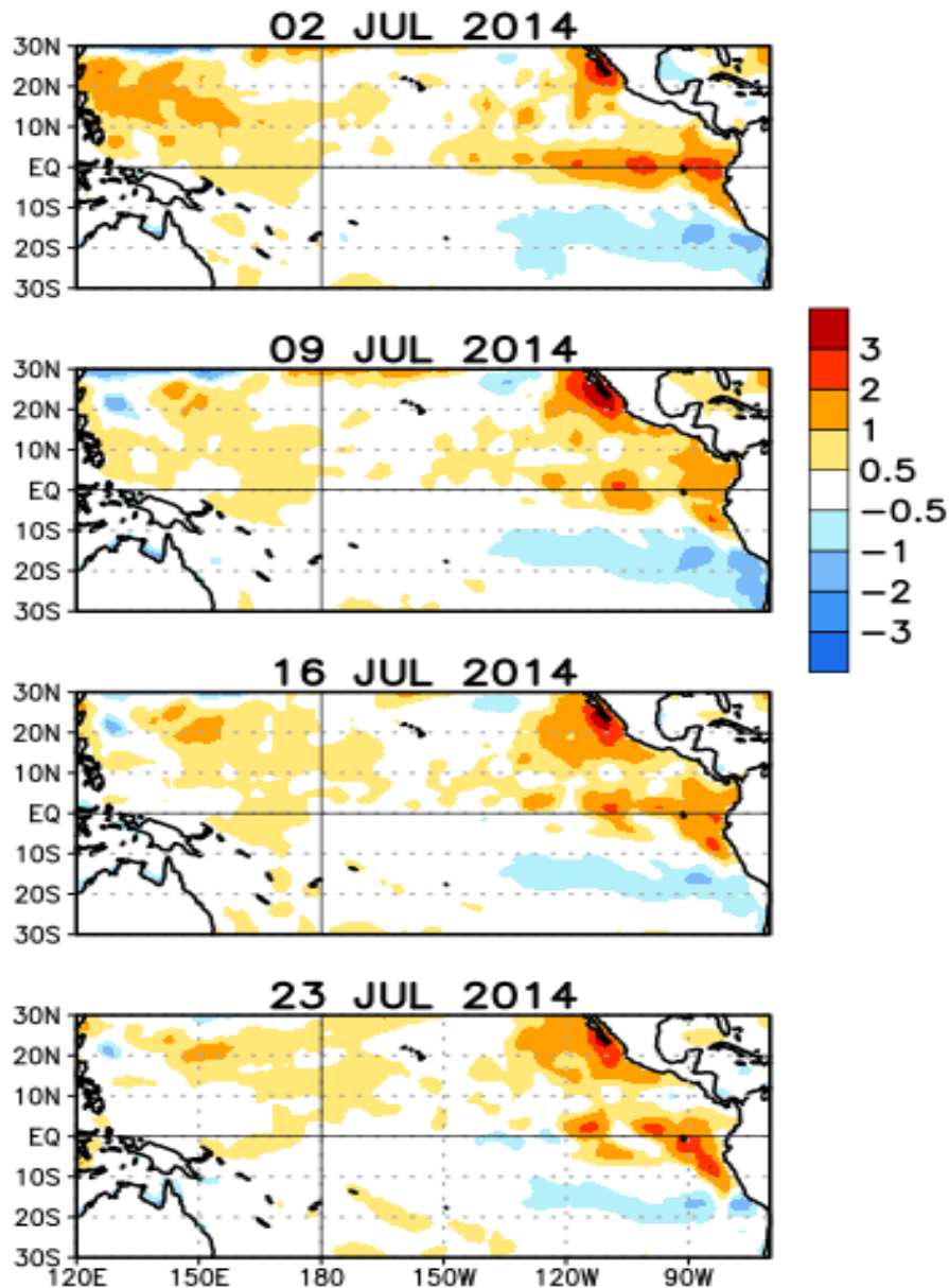
Figura 4. Anomalías de TSM para el Océano Pacífico durante las últimas cuatro semanas (°C). (Fuente: Climate Prediction Center, NOAA).
