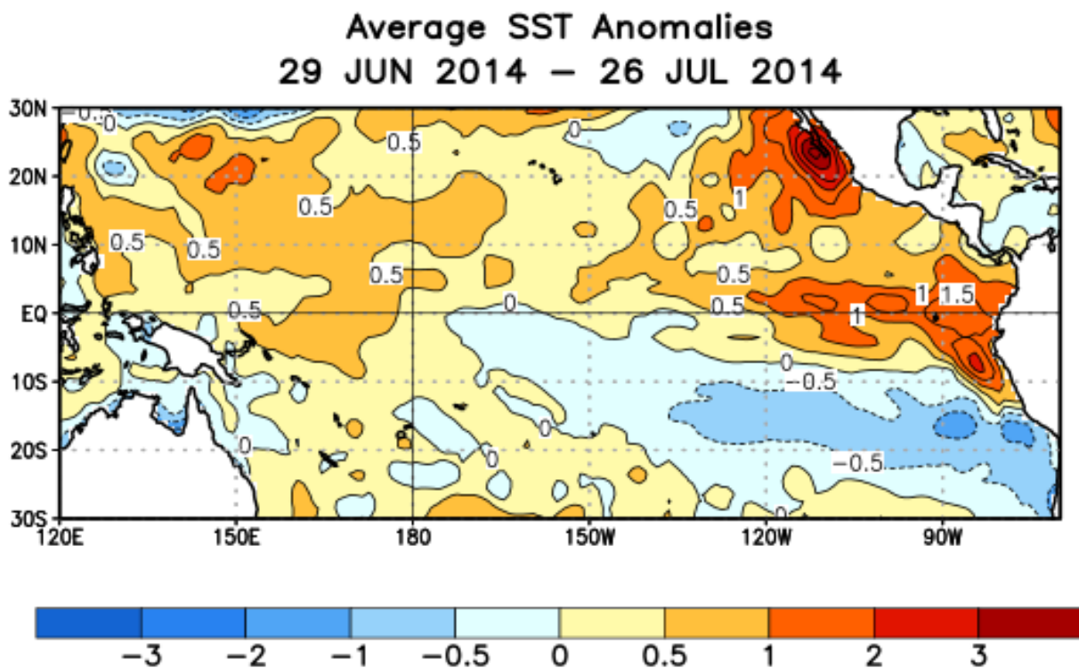
Figura 3. Anomalías de TSM en el pacifico tropical, promediadas del 29 de junio al 28 de julio de 2014 (°C). (Fuente: Climate Prediction Center, NOAA).
