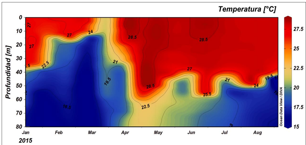
Figura 8. Serie temporal de temperatura del agua en la estación oceánica No. 5 entre 0 a 80 metros de profundidad. Período Enero – Agosto 2015 (°C) (Fuente: CCCP)
