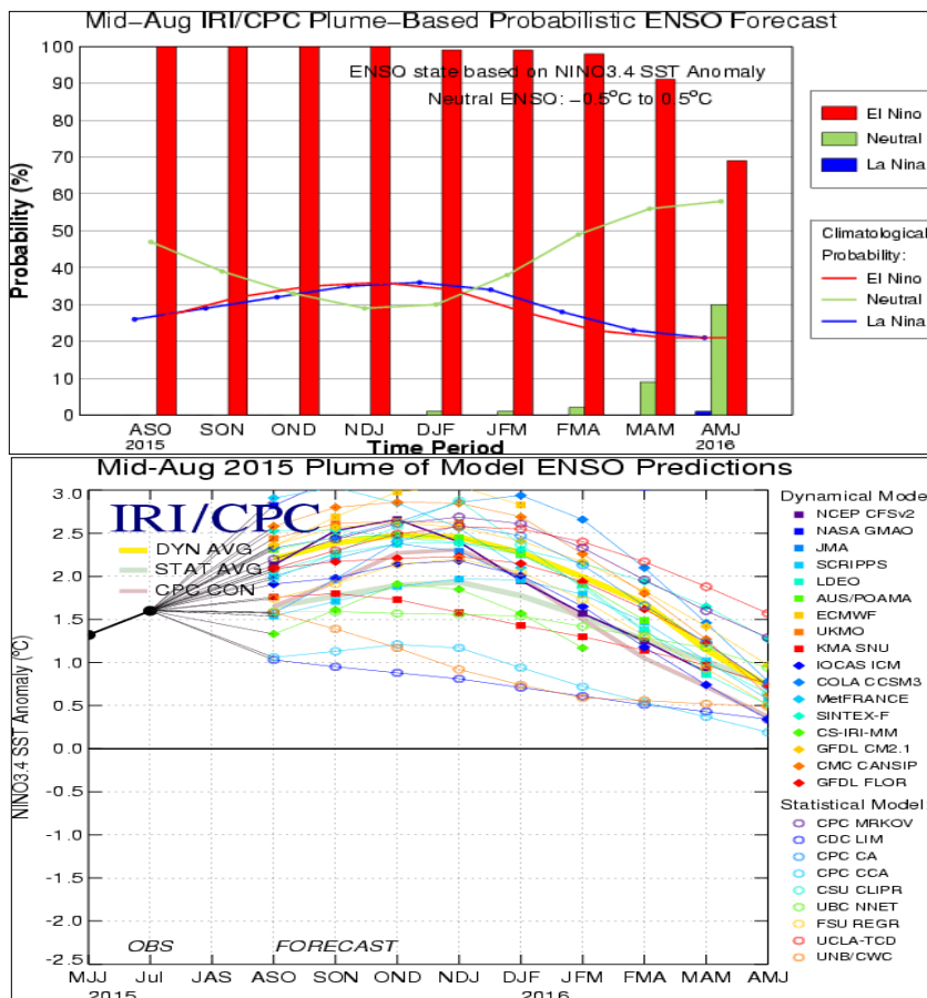
Figura 13. Pluma de salidas de los modelos estadísticos y dinámicos de predicción de condiciones ENOS agosto 20 de 2015. (Fuente: IRI/CPC).
