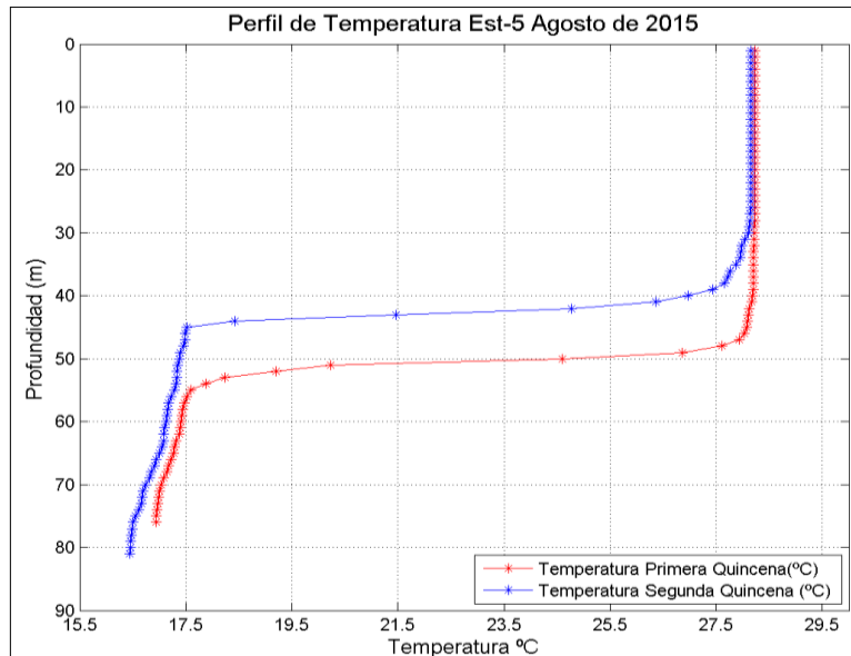
Figura 9. Perfil TSM durante el monitoreo agosto/15 en la “Estación No.5”. (Fuente: CCCP)
