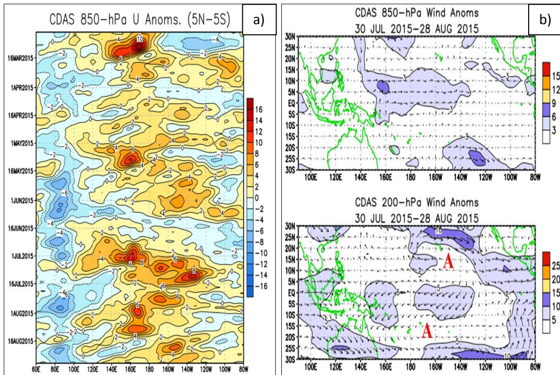
Figura 3. Anomalías en el comportamiento de los vientos sobre el Océano Pacífico Ecuatorial Agosto 2015. (Fuente: Climate Prediction Center, NOAA).
