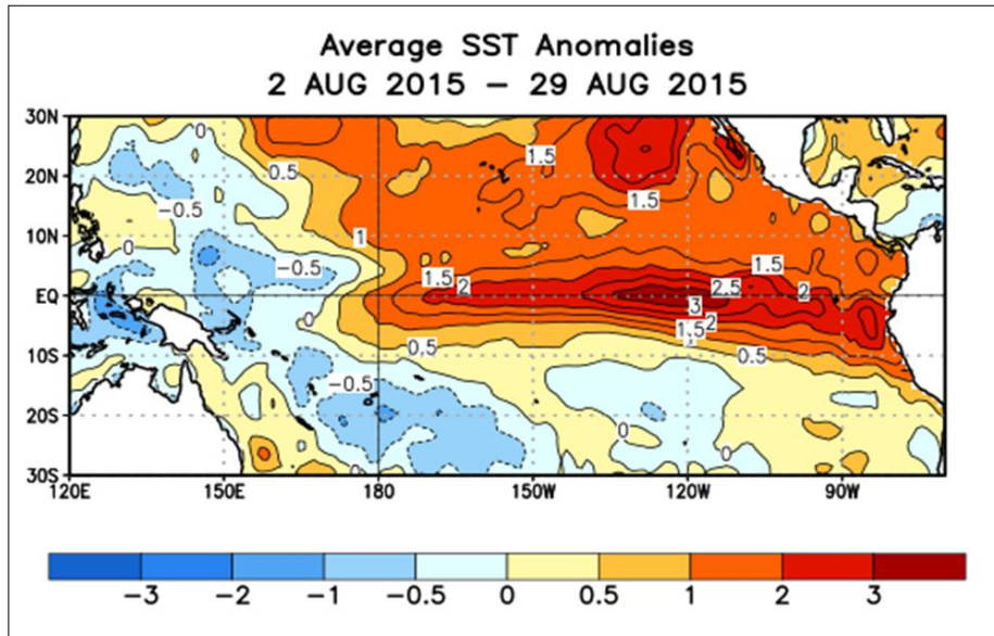
Figura 5. Anomalías de TSM en el pacífico tropical, promediadas del 02 al 29 de agosto 2015 (°C). (Fuente: Climate Prediction Center, NOAA).
