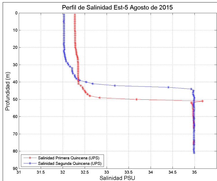
Figura 11. Perfil de la salinidad del agua durante el monitoreo agosto/15 en la “Estación No.5”. (Fuente: CCCP)
