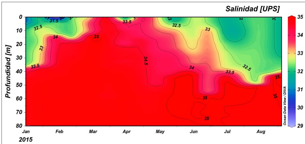
Figura 10. Serie temporal salinidad del agua en la estación oceánica No. 5 entre 0 a 80 metros de profundidad. Período Enero – agosto 2015 (UPS) (Fuente: CCCP)
