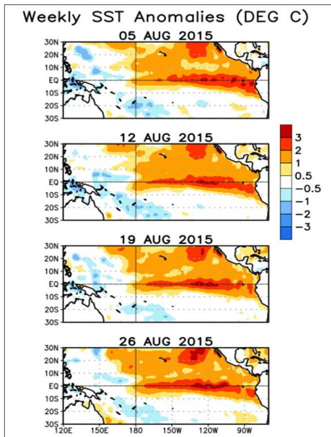
Figura 6. Anomalías de TSM para el Océano Pacífico durante las últimas cuatro semanas de agosto 2015 (°C). (Fuente: Climate Prediction Center, NOAA).
