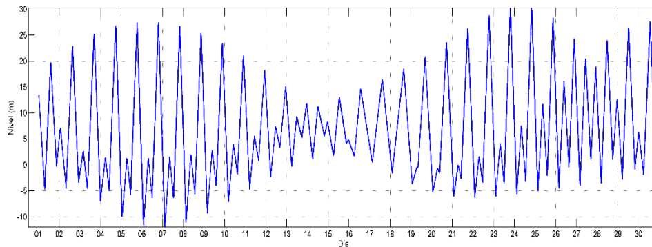
Figura 14. Pronóstico de marea para Septiembre de 2015, Cartagena. (Torres Parra & Otero Diaz, 2008)
