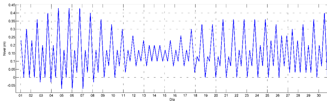
Figura 16. Pronostico de marea para septiembre de 2015 en Santa Marta. (Ideam, 2015)
