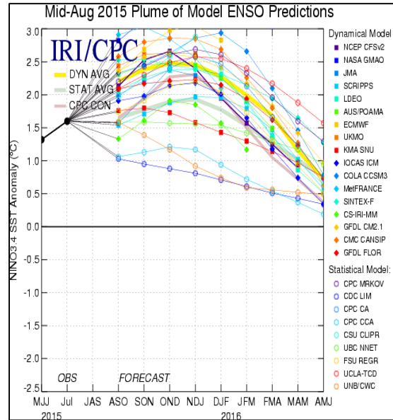
Figura 3. Pronóstico ENSO (Fuente: (IRI/CPC, 2015)).
