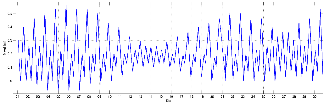
Figura 15. Pronóstico de marea para Septiembre de 2015 en (Puerto Colombia) Barranquilla. (Ideam, 2015)
