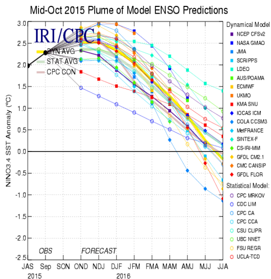
Figura 3. Pronóstico ENSO (Fuente: (IRI/CPC, 2015)).
