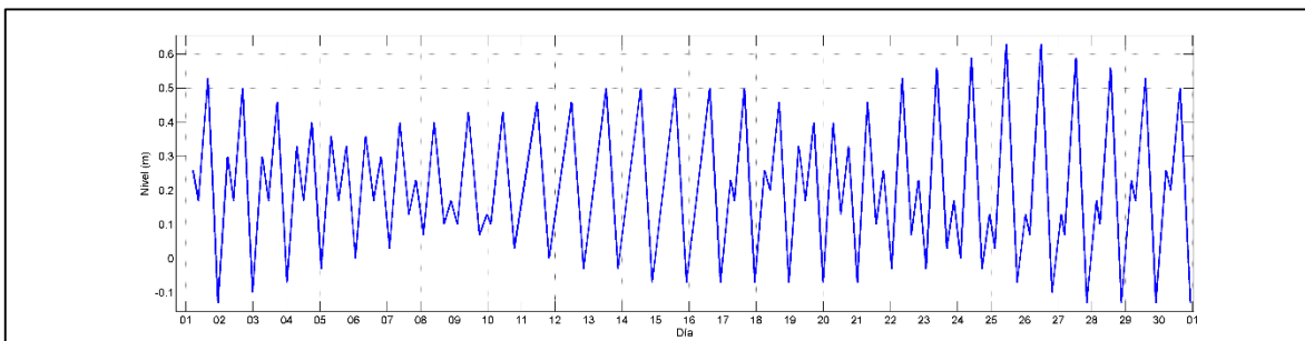
Figura 16. Pronostico de marea para noviembre de 2015 en Santa Marta. (Ideam, 2015)
