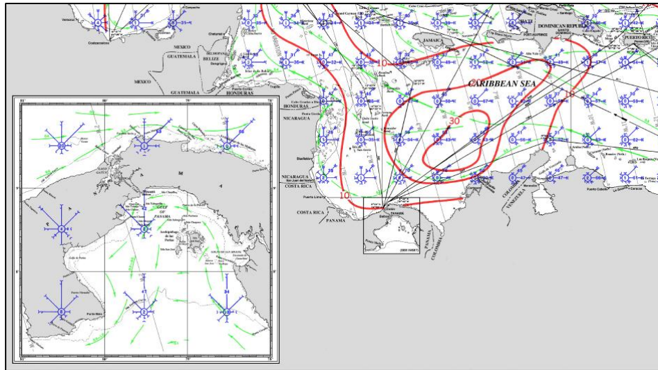
Figura 9. Climatología oceánica para el mes de Diciembre. (NGA, 2006)
