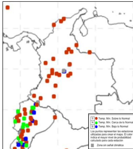
Figura 10. Pronóstico temperatura mínima para Diciembre de 2015 (Fuente: (CIIFEN, 2015)).
