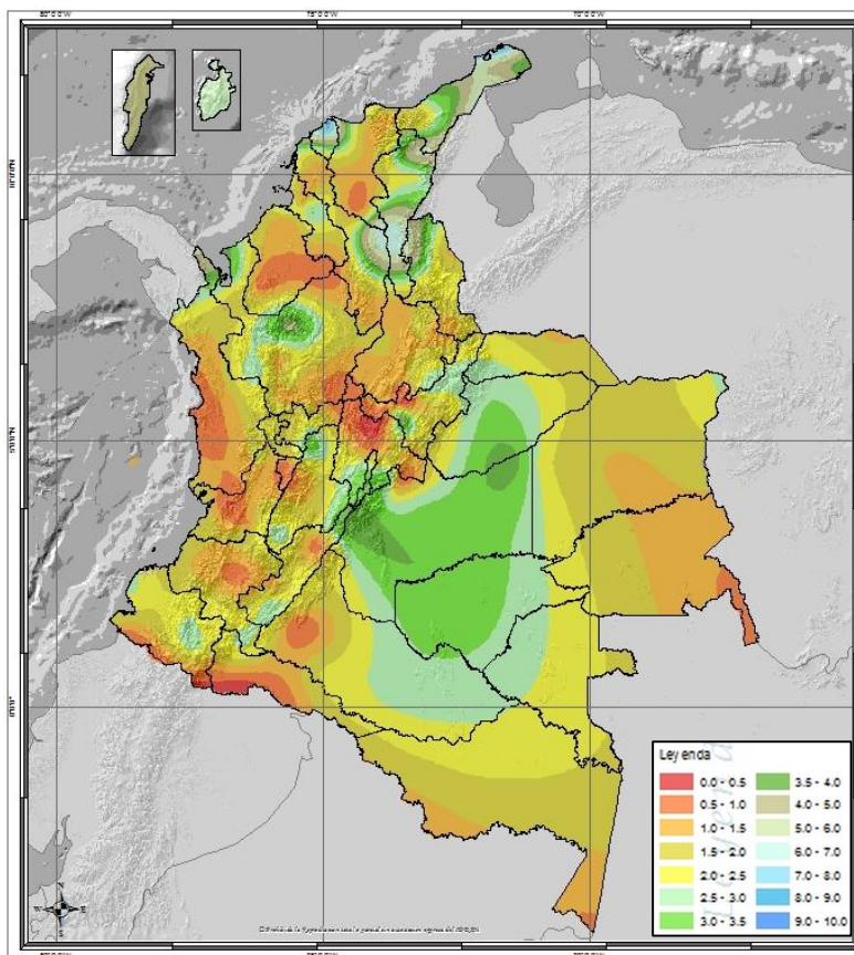
Figura 8. Velocidad del viento promedio mes de Diciembre (m/s) (continente). (Ideam)
