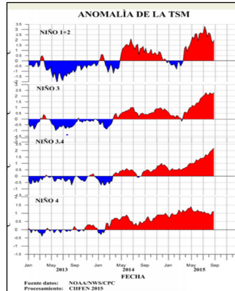
Figura 2. Anomalías TSM en cada una de las regiones de "El Niño" (Fuente: (CPC-NCEP, 2015)).
