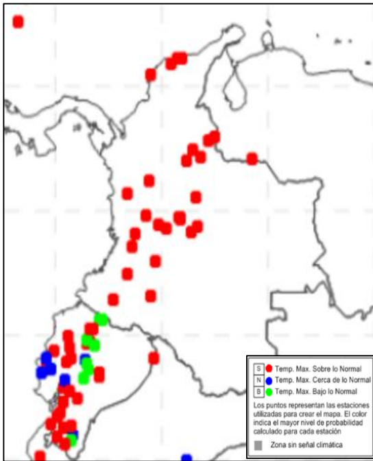
Figura 9. Pronóstico temperatura máxima para Diciembre de 2015 (Fuente: (CIIFEN, 2015)).
