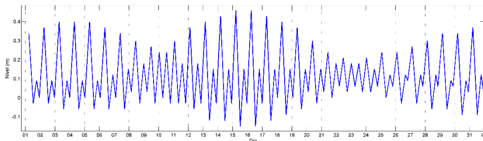
Figura 15. Pronóstico de marea para Marzo de 2016 en (Puerto Colombia) Barranquilla. (Ideam, 2016)
