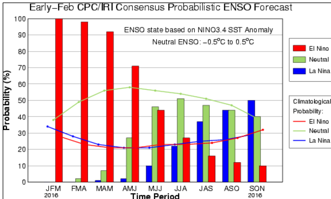
Figura 4. Pronóstico de las condiciones ENSO esperadas para el lapso enero de 2016 hasta noviembre de 2016 (Fuente: (IRI/CPC, 2016)).
