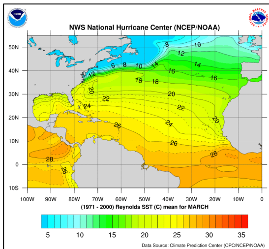
Figura 12. Pronóstico de TSM para Marzo de 2016 (Fuente: (NHC, 2016)).
