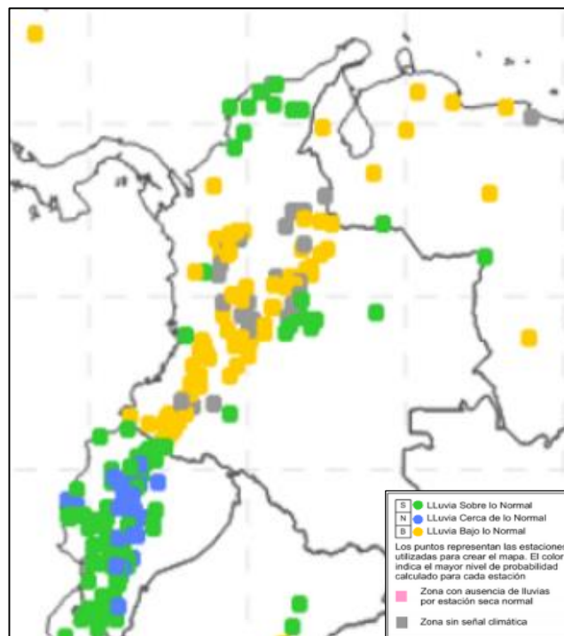
Figura 5. Pronóstico de precipitación para el mes de Marzo de 2016 (Fuente: (CIIFEN (. I., 2016)).
