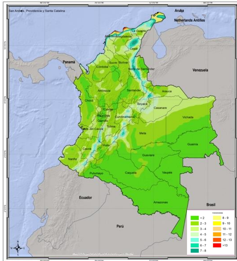
Figura 8. Velocidad del viento promedio mes de Marzo (m/s) (continente). (Ideam)
