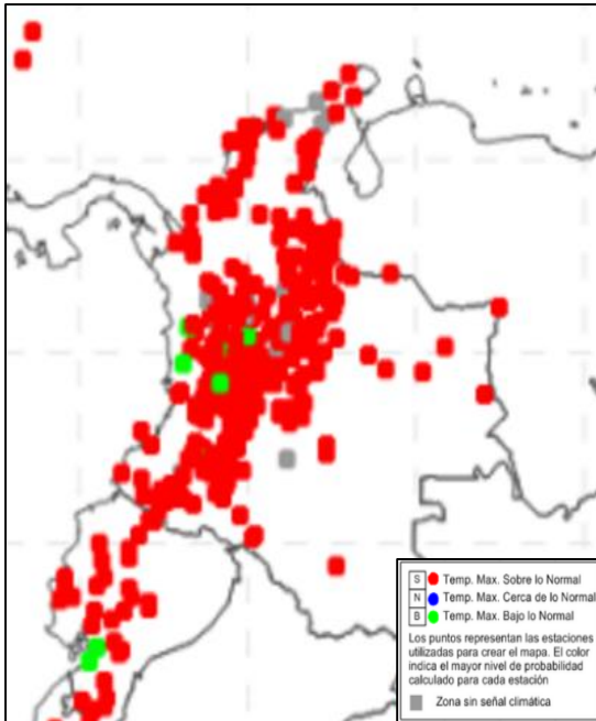
Figura 9. Pronóstico temperatura máxima para Marzo de 2016 (Fuente: (CIIFEN (. I., 2016)).
