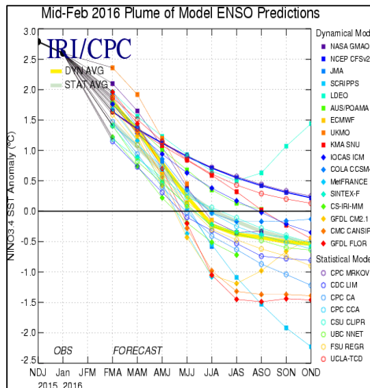
Figura 3. Pronóstico ENSO (Fuente: (IRI/CPC, 2016)).
