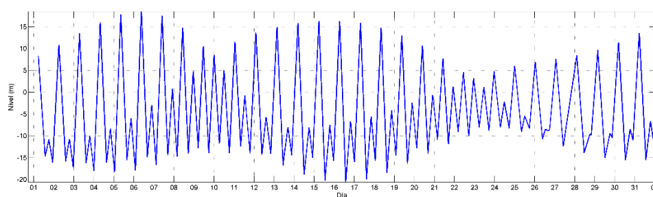
Figura 14. Pronóstico de marea para Marzo de 2016, Cartagena. (Torres Parra & Otero Diaz, 2008)
