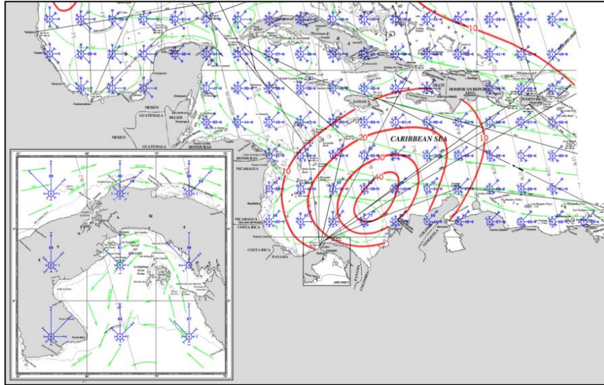
Figura 11. Climatología oceánica para el mes de Marzo. (NGA, 2006)
