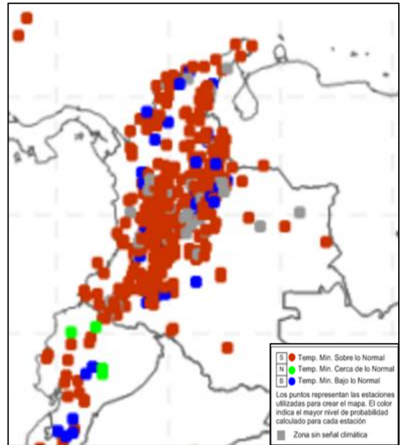
Figura 10. Pronóstico temperatura mínima para Marzo de 2016 (Fuente: (CIIFEN (. I., 2016)).
