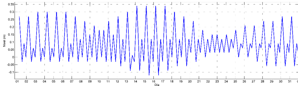
Figura 16. Pronostico de marea para Marzo de 2016 en Santa Marta. (Ideam, 2016)
