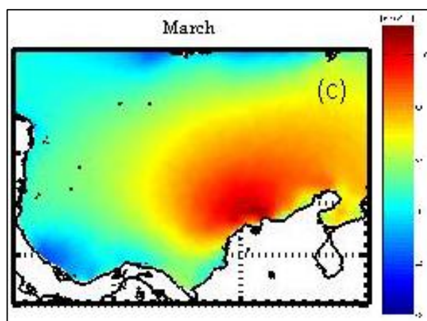
Figura 6. Promedio multianual velocidad del viento (m/s) mes de Marzo. (Appendini, 2014)
