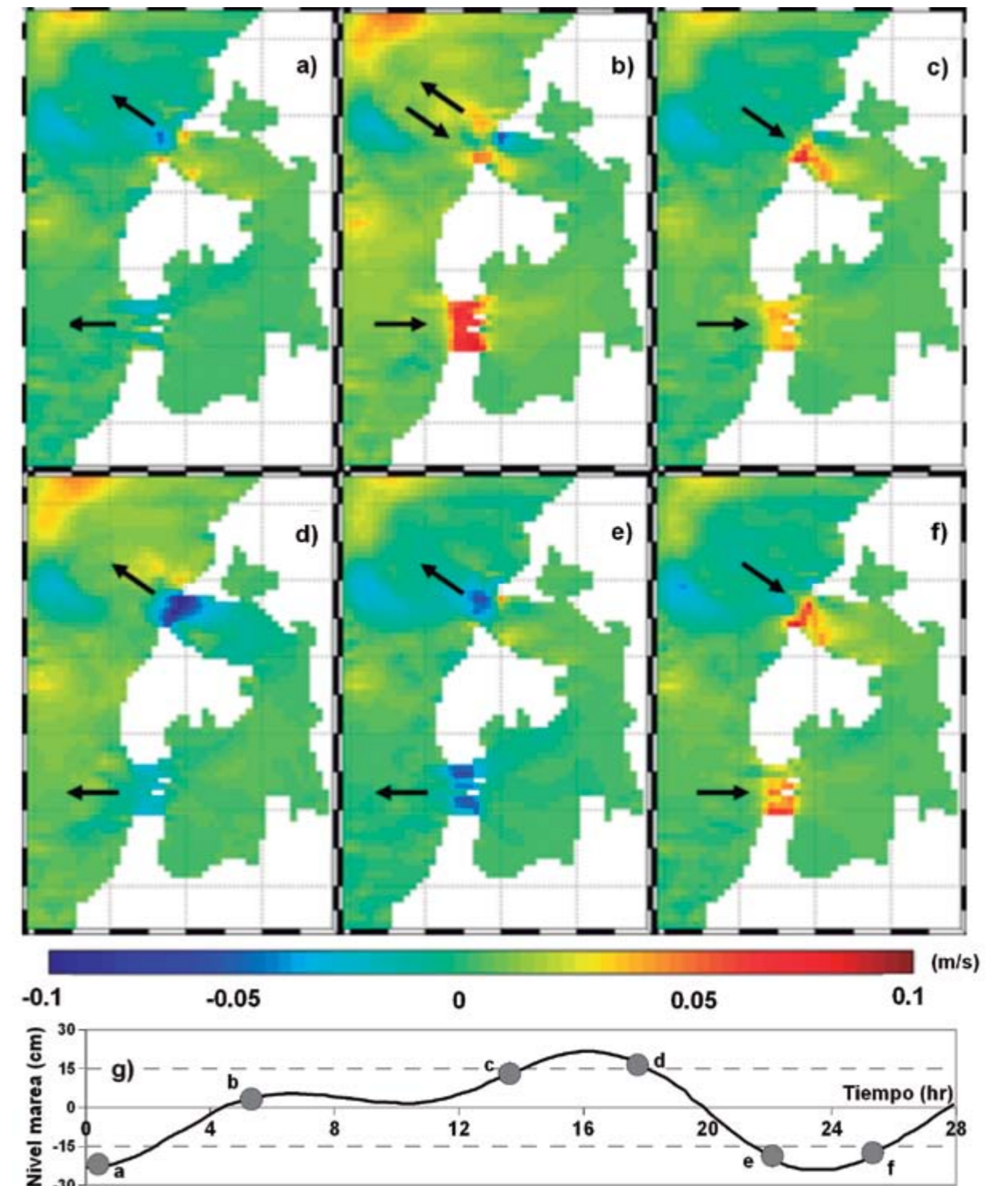
Figura 5. De a) a f) se muestra el componente u de la corriente promediado e integrado verticalmente (no se considera la descarga del Canal del Dique). En g) se grafica el correspondiente estado de la marea para cada uno de los regímenes de corrientes; los puntos grises indican la hora a la cual la correspondiente corriente, verticalmente integrada, fue obtenida. Las flechas representan la corriente de flujo y reflujo.
