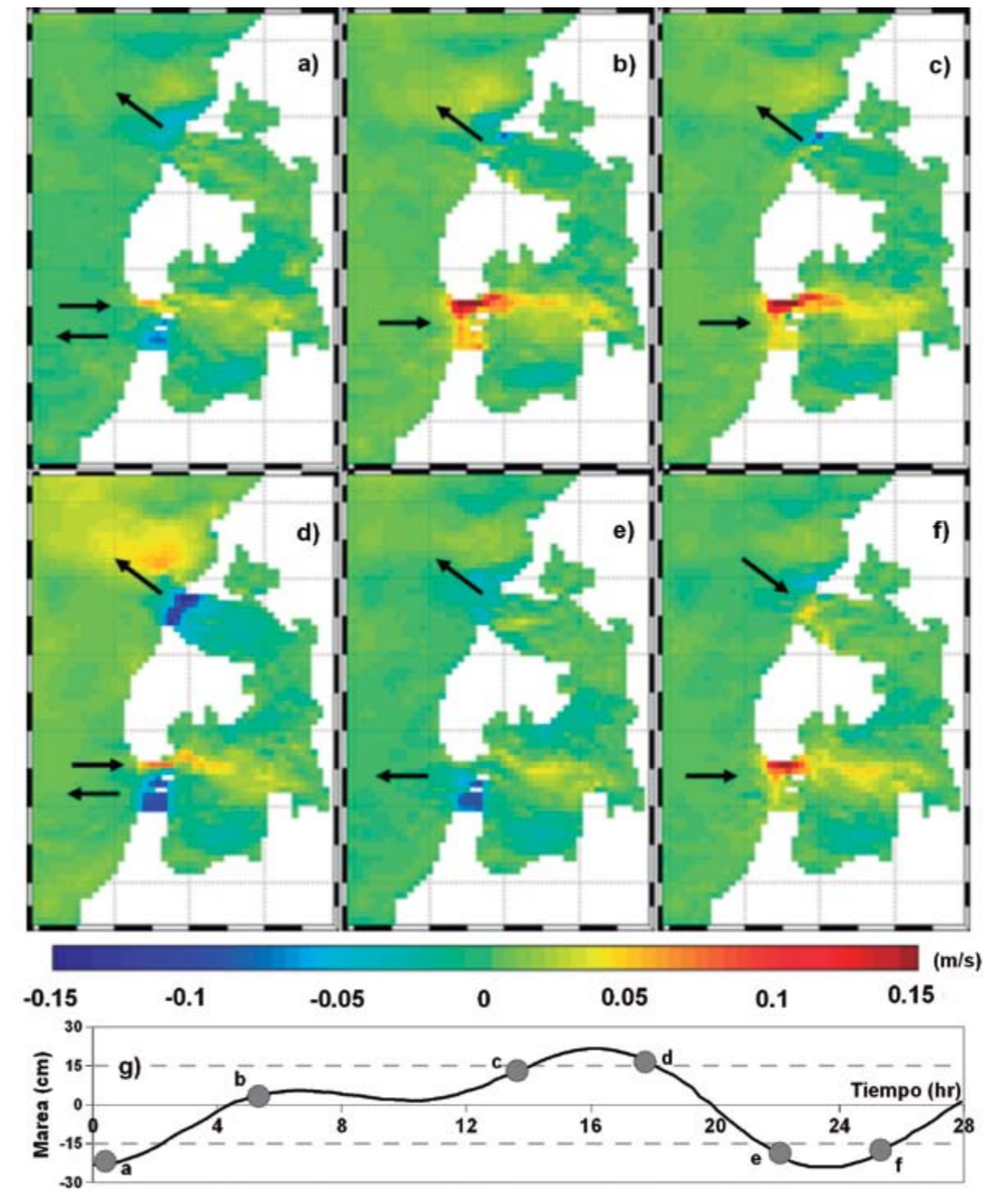
Figura 10. De a) a f) se muestra el componente u de la corriente promediado e integrado verticalmente, teniendo en cuenta la baja descarga del Canal del Dique (BDCD- 50 \text{ m}^3/\text{s} ). En g) se grafica el ciclo de la marea empleado; los puntos grises indican la hora a la cual corresponde el patrón de corrientes graficadas de a) a f) ; las flechas representan las corrientes de flujo y refluo.
