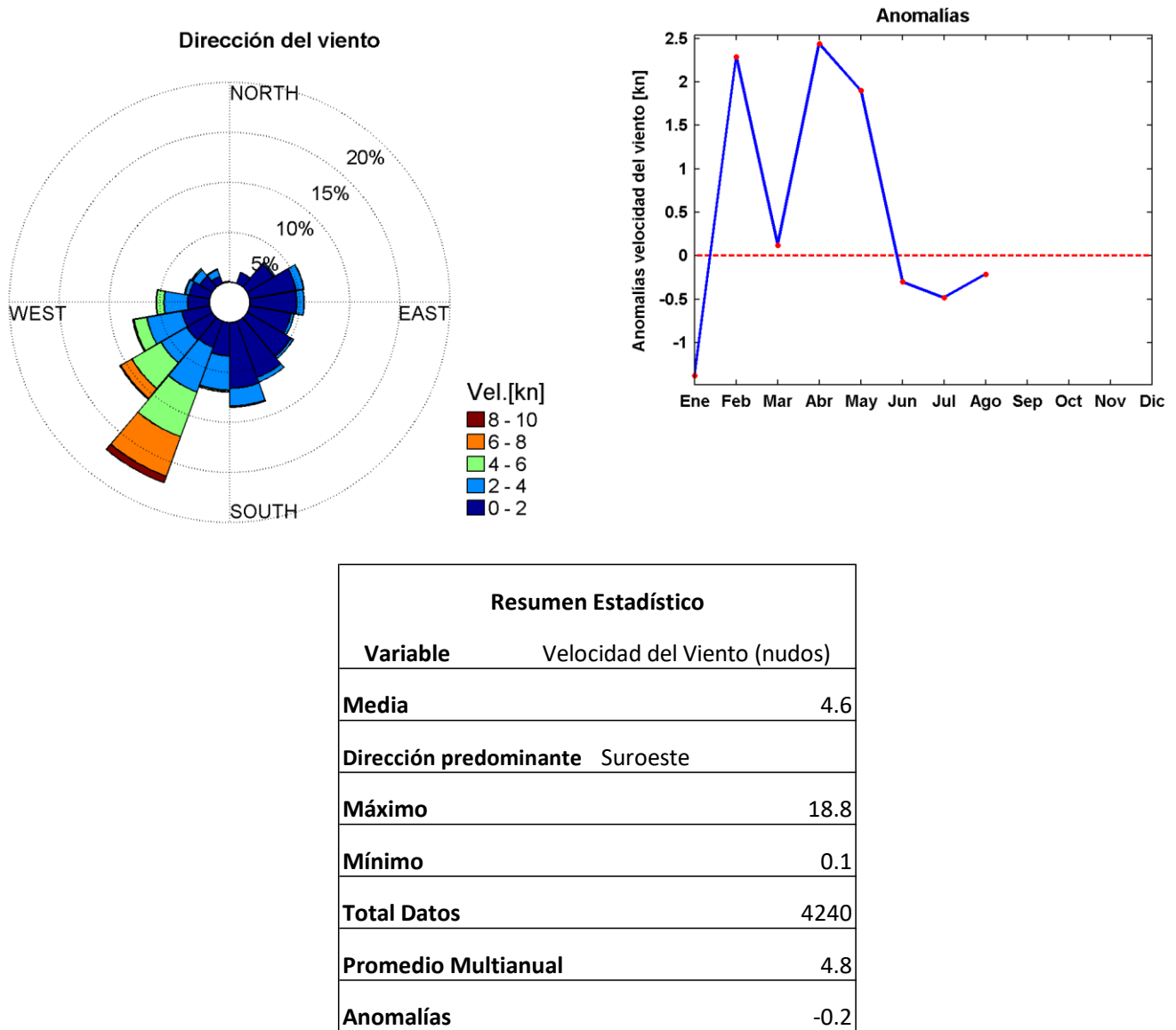
Figura 11. Distribución de frecuencia de la dirección, velocidad, anomalía velocidad y resumen estadístico del viento en Buenaventura.
